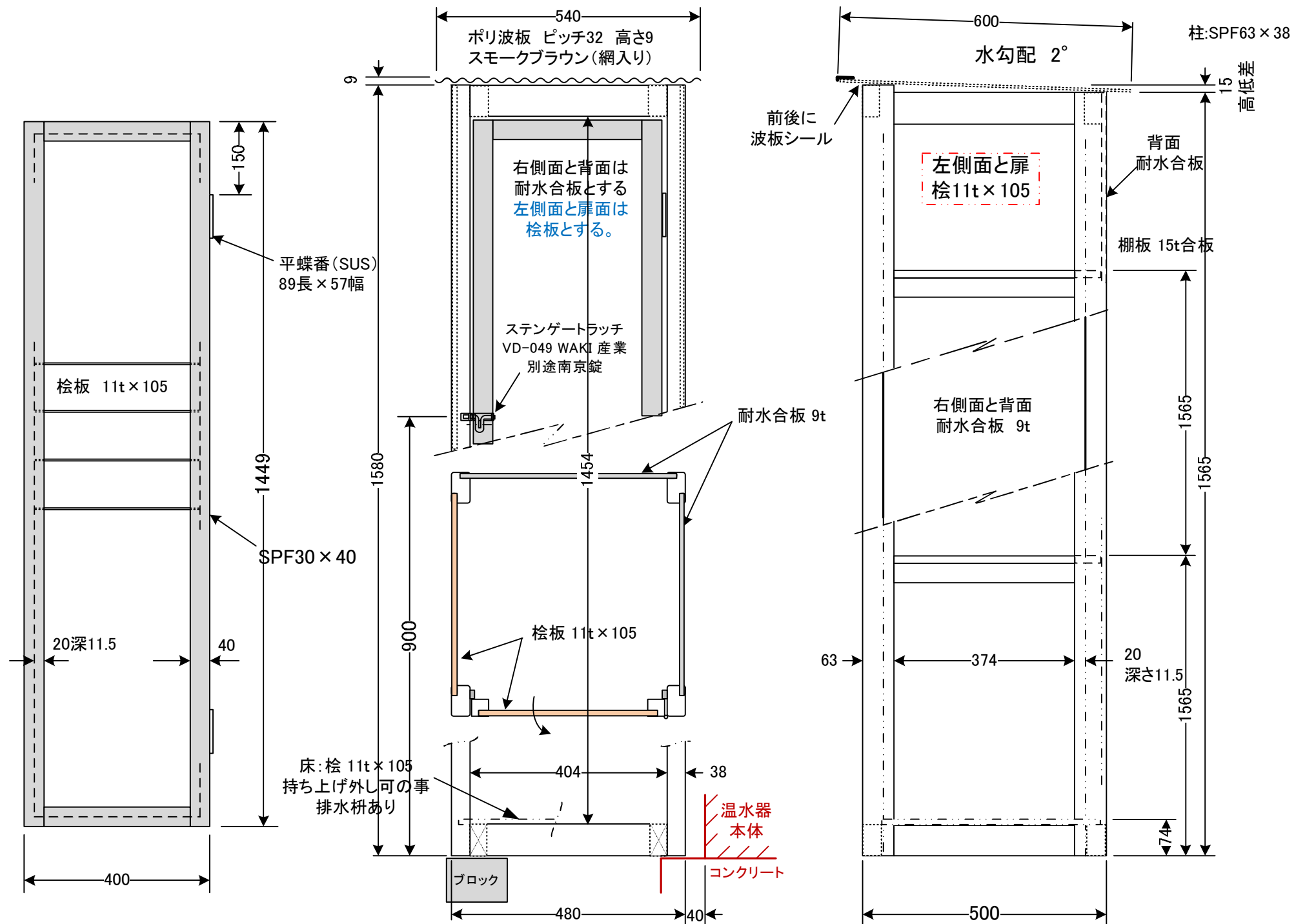
扉正面図
